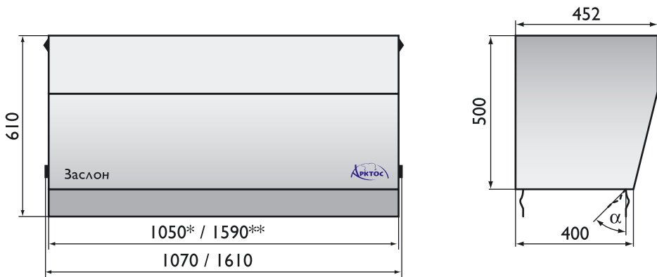
Общий вид завес «Заслон»
